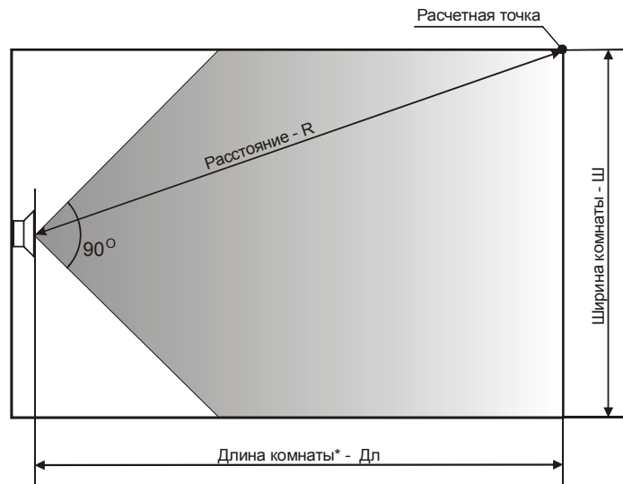
Рис. 4 . Расположение оповещателя по центру «Комнаты».
