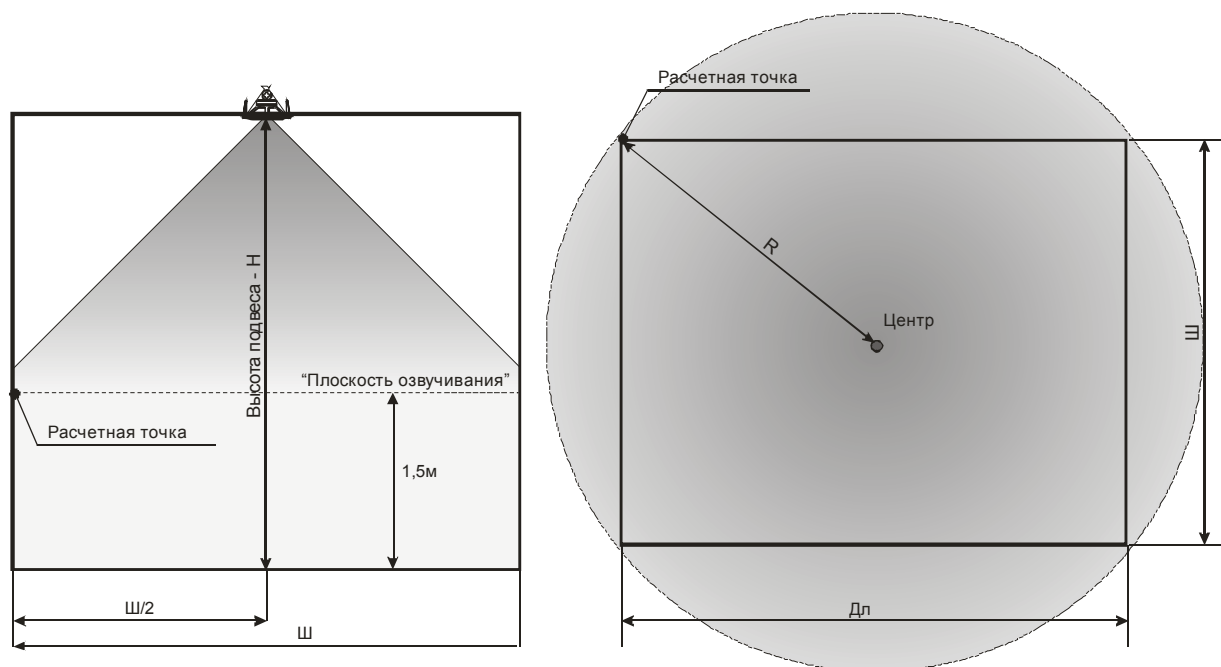
Рис 6. Плоскость озвучивания при высоких потолках, «расчётная точка» выше 1.5 м.
