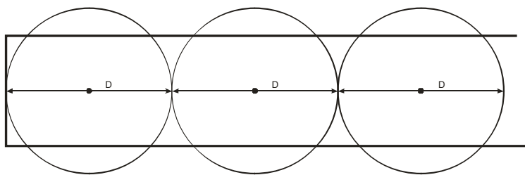
Рис.25. Размещение оповещателей в помещении типа «Коридор» при высоте потолка более 4-х метров и расстояние «до расчётной точки».
