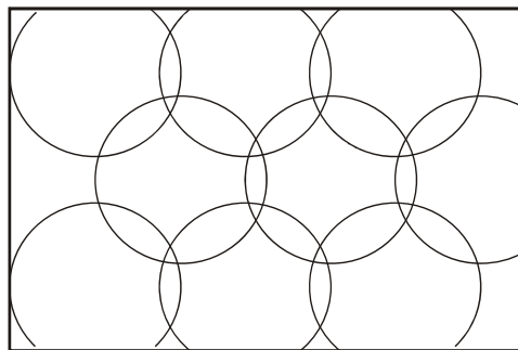
Рис. 22. Пример размещения оповещателей.
