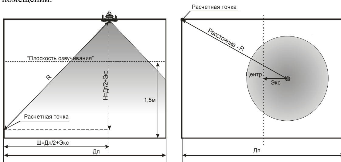
Рис. 8. Расположение потолочного оповещателя со смещением (эксцентриситетом) от геометрического центра «Комнаты».
