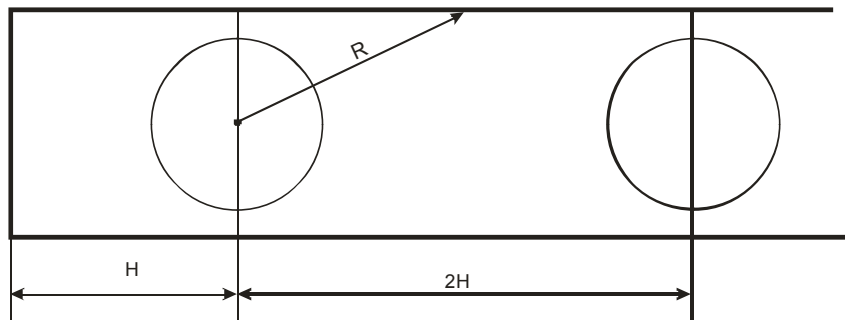
Рис. 27. Размещение оповещателей в помещении типа «Коридор» при высоте потолка ниже 3,5 метров (горизонтальная проекция).
