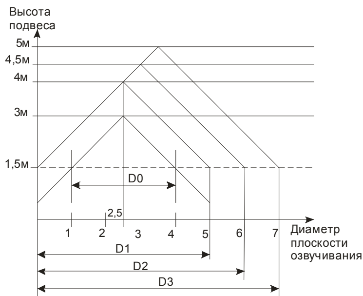
Рис.20. График зависимости диаметра плоскости озвучивания от высоты потолка.
