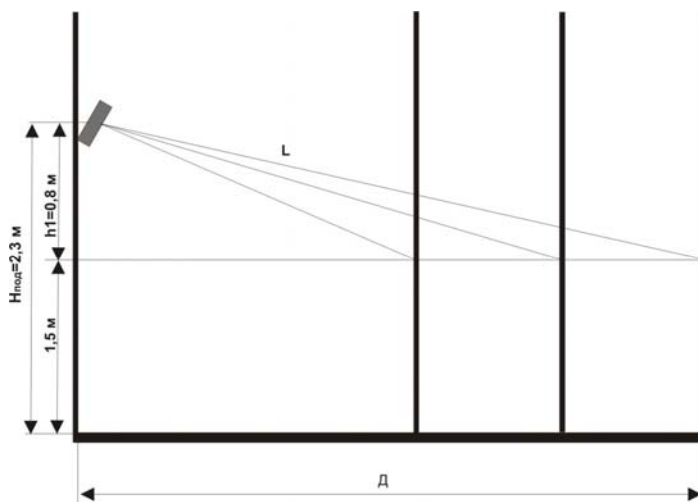
Рис. 3. Вертикальная проекция крепления настенного оповещателя по НПБ.
