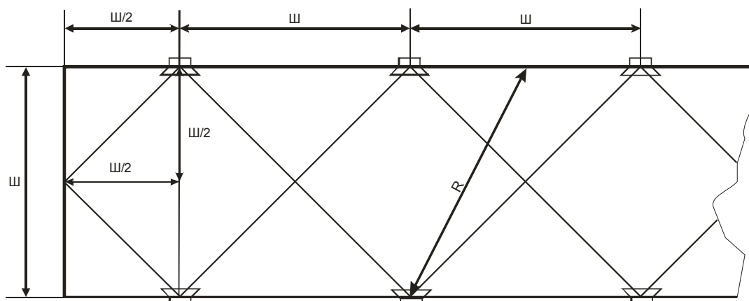
Рис. 18. Размещение оповещателей в помещении типа Малый «Зал» формы «Прямоугольник» и положение «расчётной точки».
