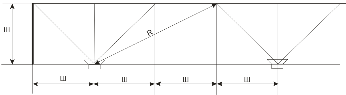
Рис.23. Размещение оповещателей в помещении типа «Коридор» при ширине менее 3-х метров и расстояние «до расчётной точки».
