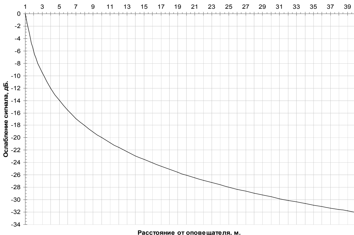
График ослабления звукового сигнала F(R)=20*\lg(1/R)
