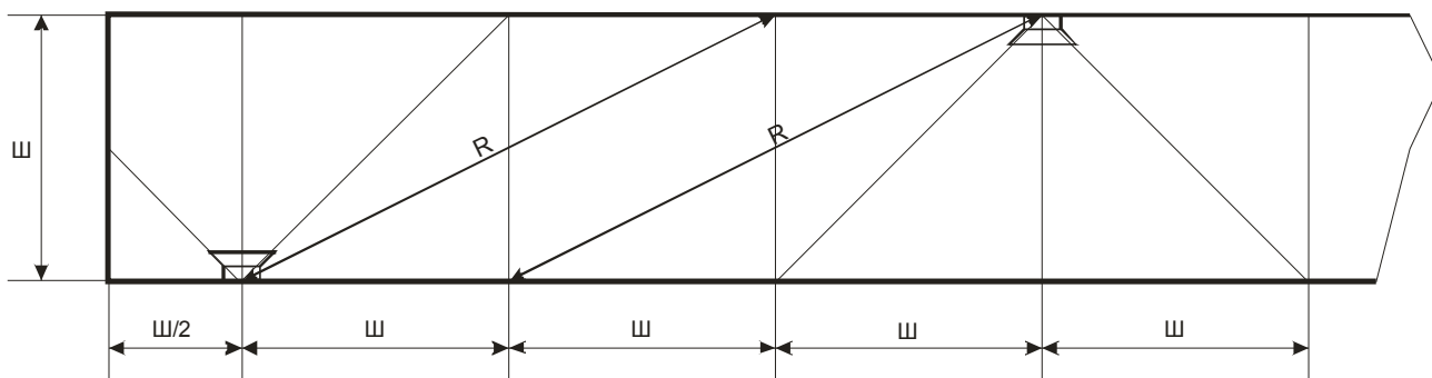
Рис.24. Размещение оповещателей в помещении типа «Коридор» при ширине более 3-х метров и расстоянии «до расчётной точки».
