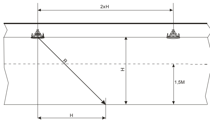
Рис.26. Размещение оповещателей в помещении типа «Коридор» при высоте потолка ниже 3,5 метров и расстояние «до расчётной точки» (вертикальная проекция).
